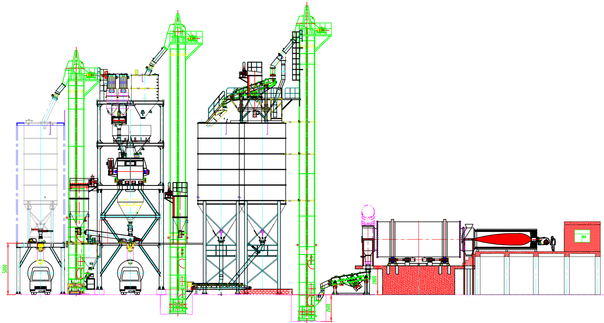
设备展开图
