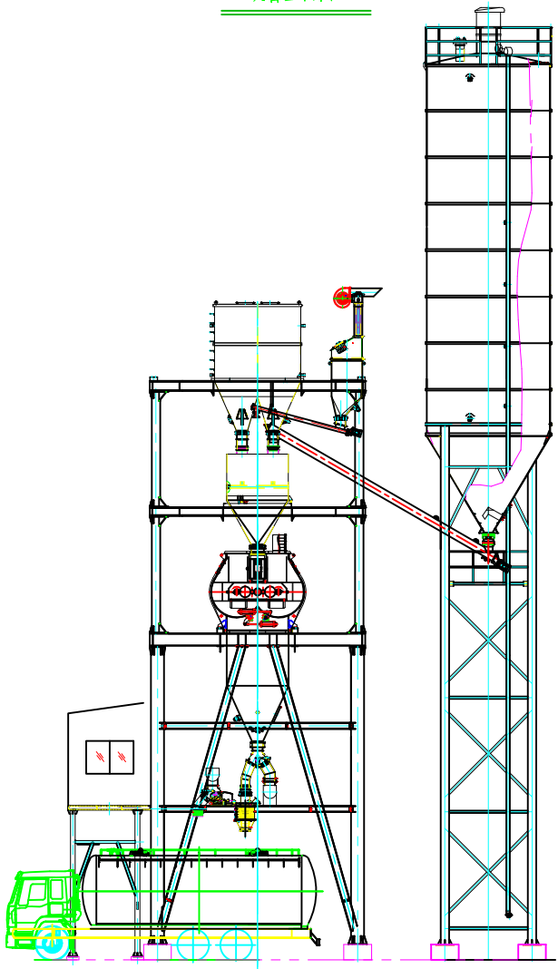
设备立面图
